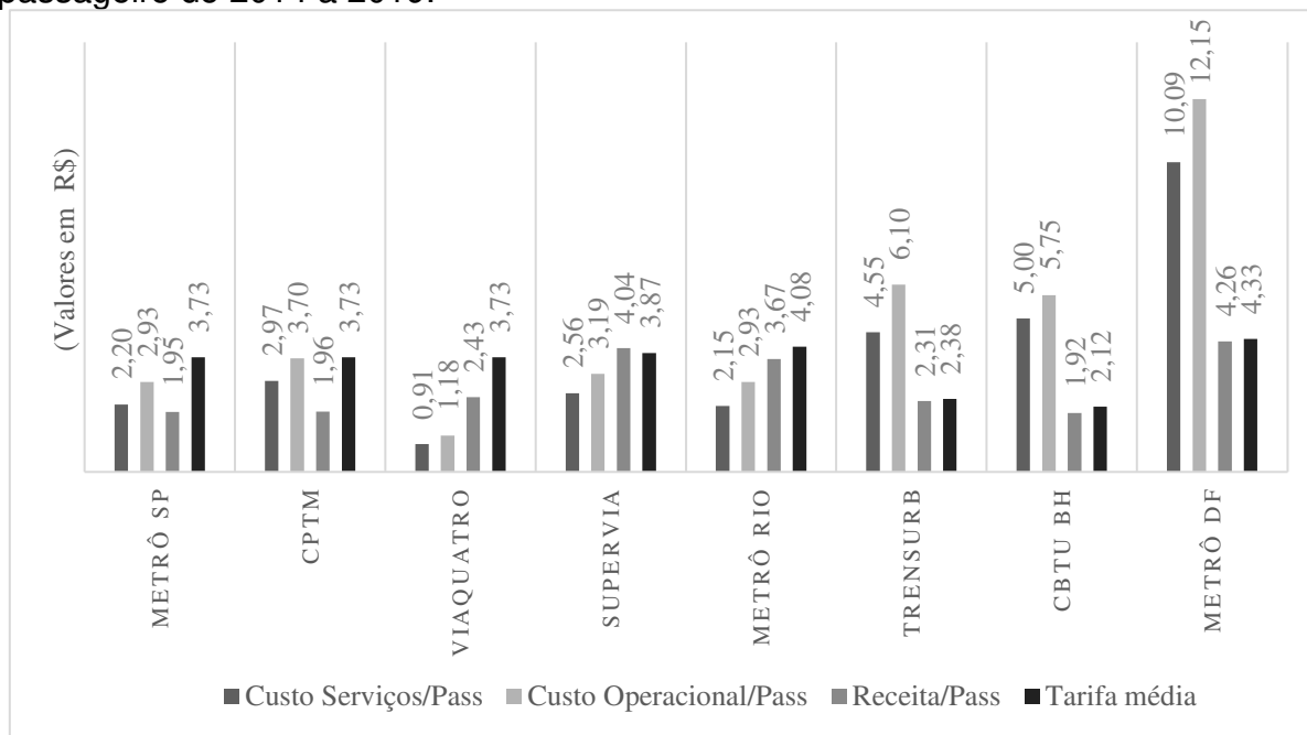
Figura 4. Custos, receitas e tarifas médias de 2014 - 2019
